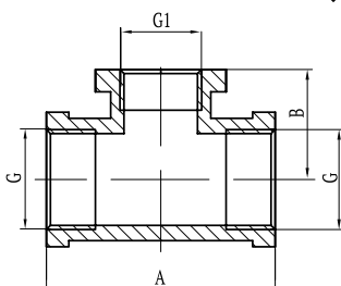
Тройник переходной вн/вн/вн VRT
