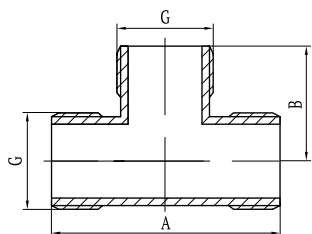
Тройник переходной вн/вн/вн VRT
